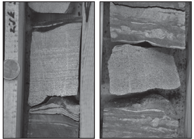
Vrtná jádra paleogenních hornin z vrtu Krumvíř 1Ra, hloubka 3 320 m.
