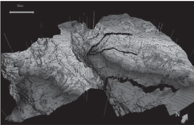
Ukázka interpretace geologické stavby nesvačilského příkopu z 3D seismických dat
